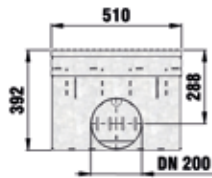
Sumidero con cestillo galvanizado
